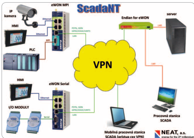
Obr. Konfigurácia centrálneho SCADA systému cez VPN
